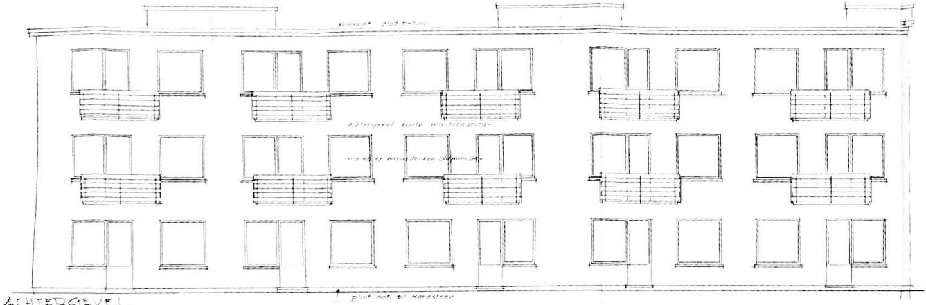
ACHTERGEVEL.
