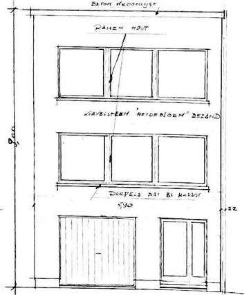
VOORGEVEL DEBUUR LOT 5
