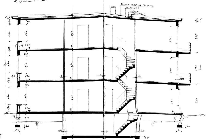
DOORSNEDEN C-D.
