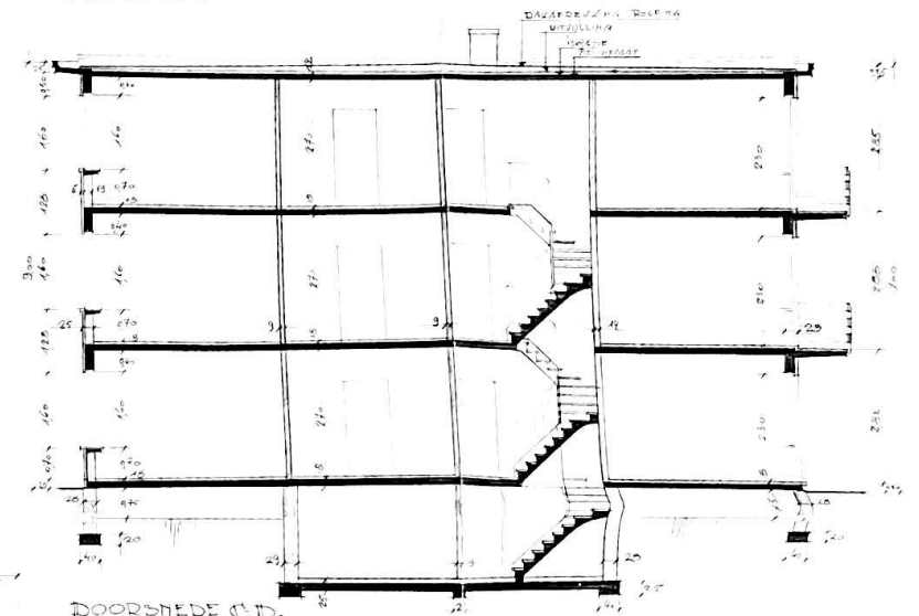
DOORSNEDEN C-D.
