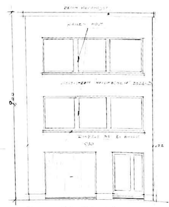
VOORGEVEL detail Lot 5
