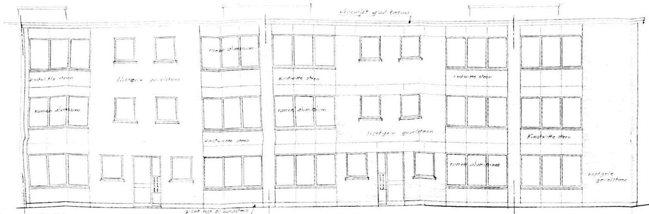
VOORGEVEL.
